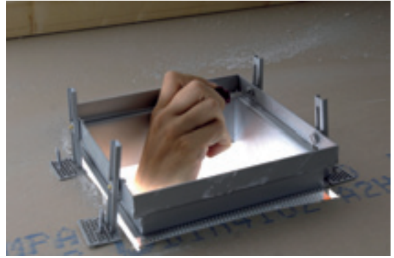
Justierung des Einbaurahmens im Deckenausschnitt und Fixierung der Position mit den vier Stellschrauben.
